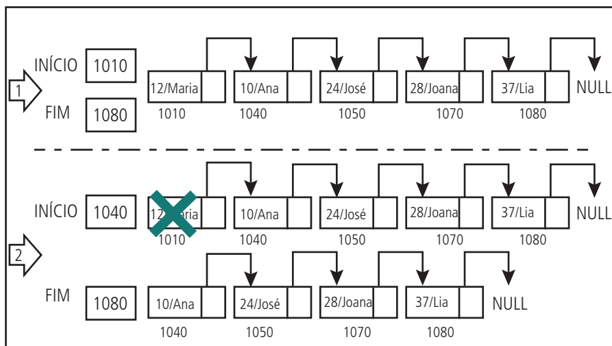
Figura 5.8: Fila dinâmica – remoção
