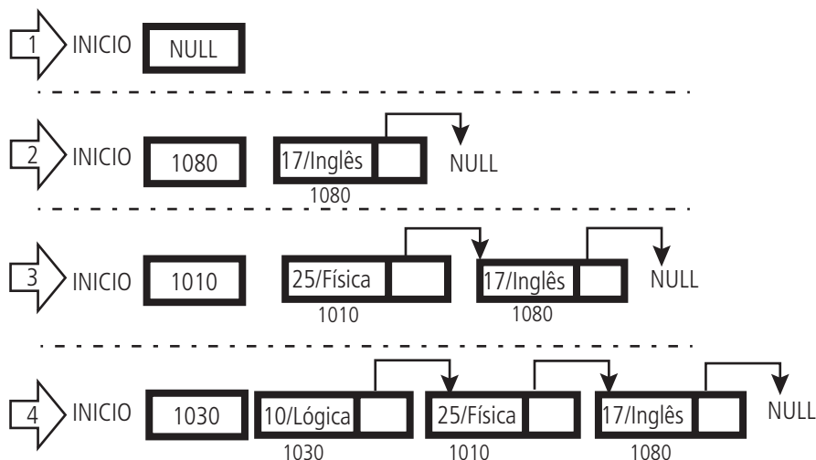
Figura 4.4: Inserção da pilha dinâmica
