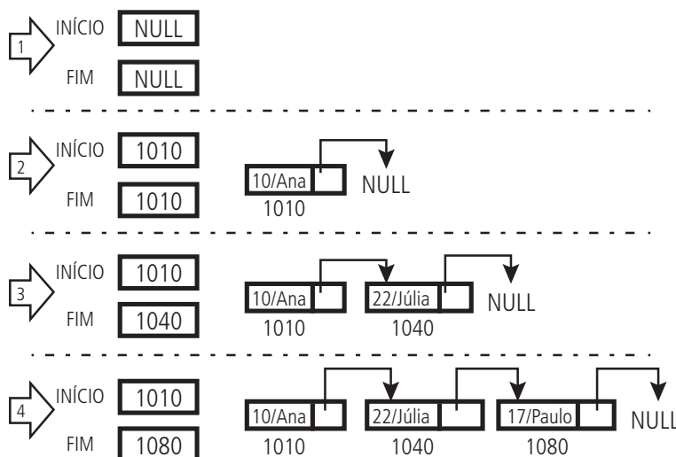
Figura 3.7: Inserção da lista dinâmica desordenada
