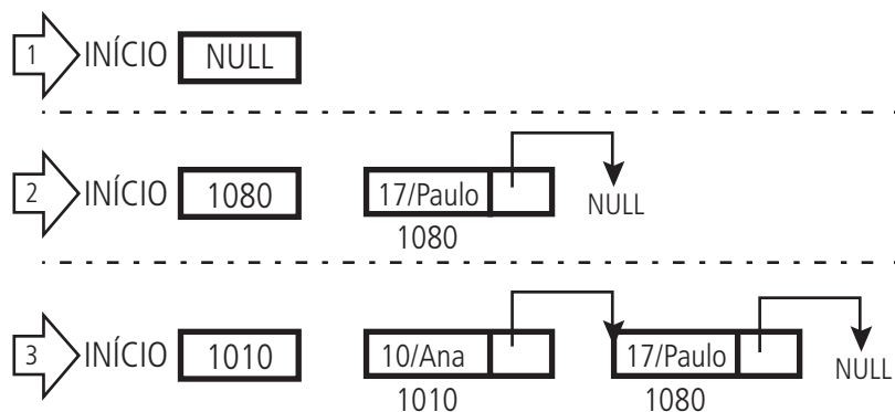
Figura 3.10a: Inserção da lista dinâmica ordenada
