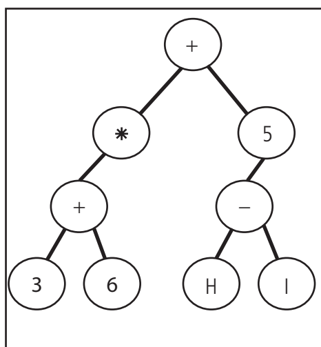
Figura 5.15: Árvore binária de expressão aritmética
