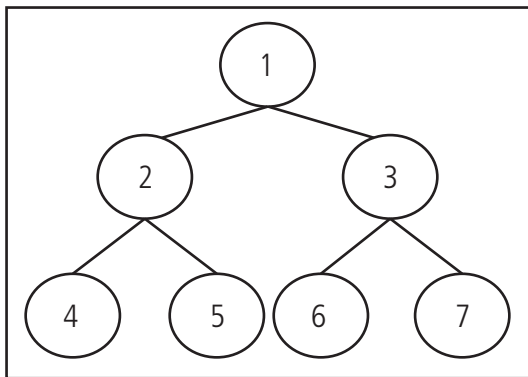
Figura 5.12: Árvore binária nível 3
