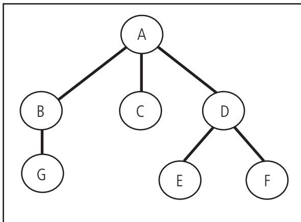
Figura 5.16: Árvore binária
