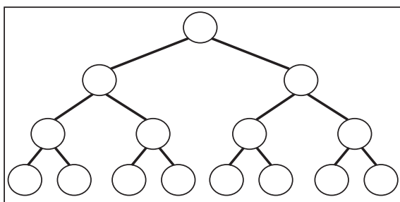
Figura 5.13: Árvore binária
