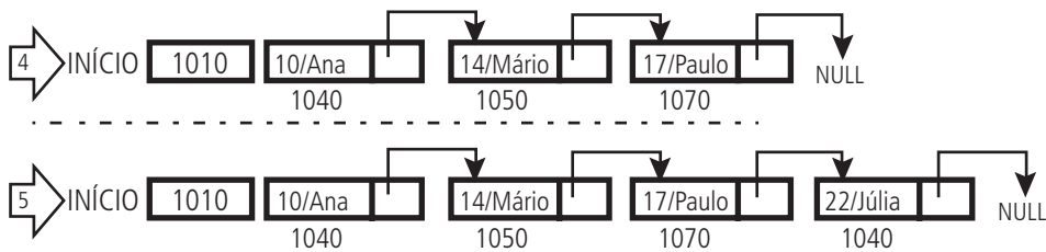
Figura 3.10b: Inserção da lista dinâmica ordenada
