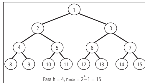
Figura 5.14: Cálculo de nós da árvore
