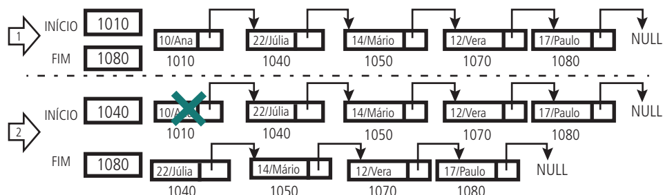
Figura 3.9a: Remoção da lista dinâmica desordenada
