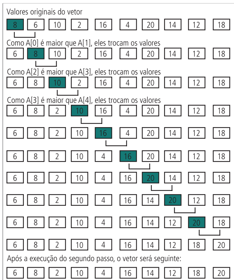
Figura 6.1: Execução do método da bolha
