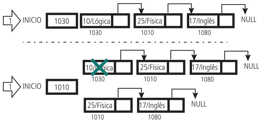
Figura 4.5: Remoção da pilha dinâmica
