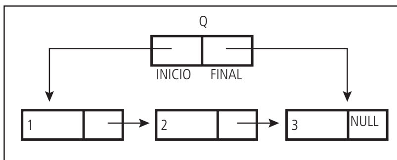
Figura 5.6: Fila dinâmica
