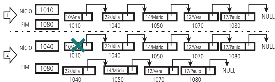
Figura 3.8: Consulta da lista dinâmica desordenada
