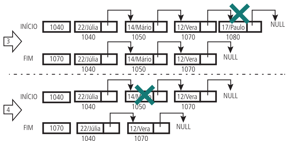
Figura 3.9b: Remoção da lista dinâmica desordenada
