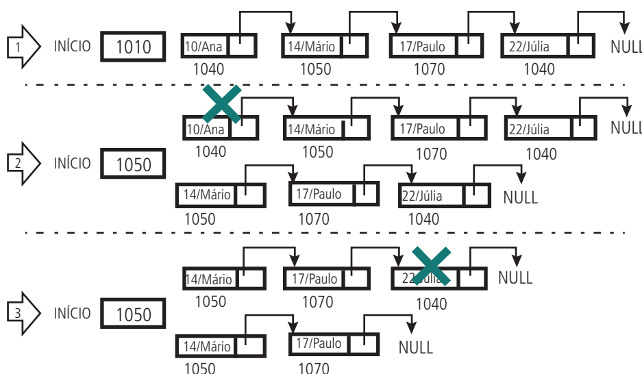
Figura 3.12: Remoção da lista dinâmica ordenada
