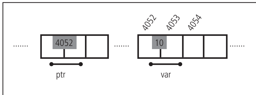
Figura 2.1: Inicialização de ponteiro
