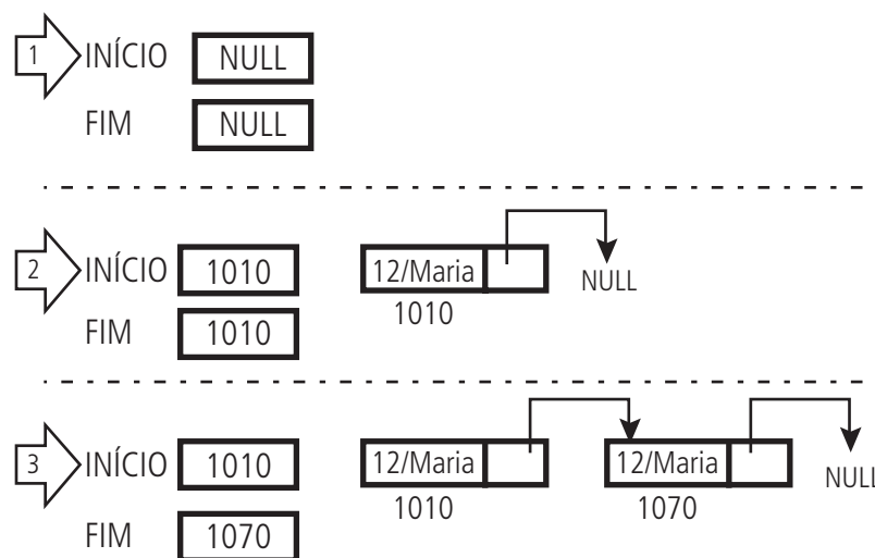
Figura 5.7: Fila dinâmica – inserção
