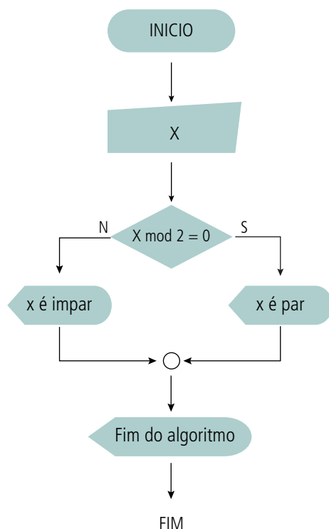
Figura 6.4: Representação do diagrama de blocos para o algoritmo par_impar
