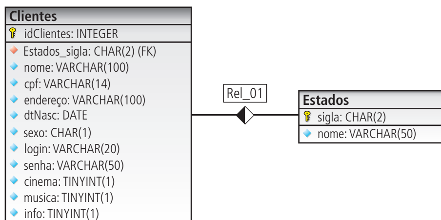
Figura 3.1: Tabelas a serem utilizadas nos exemplos
