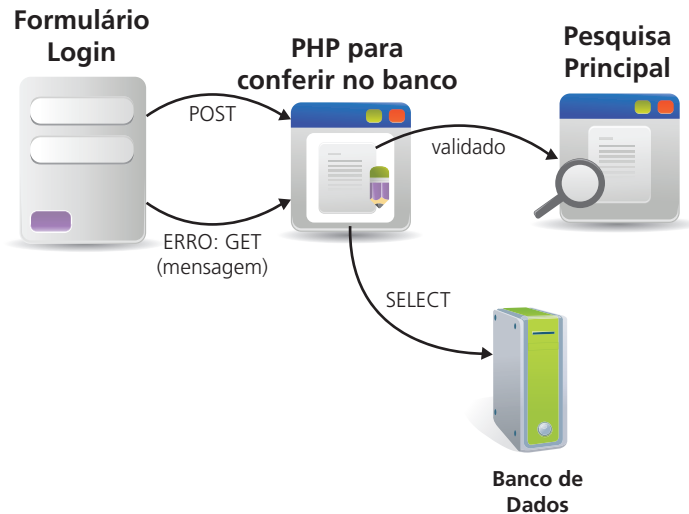
Figura 5.3: Diagrama de navegação para realizar o login
