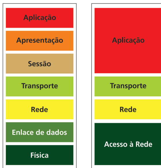
Figura 6.3 Correspondência entre camadas do modelo OSI e TCP/IP
