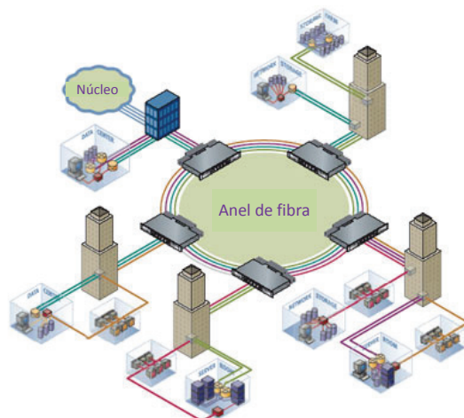
Figura 2.4 Redes metropolitanas
