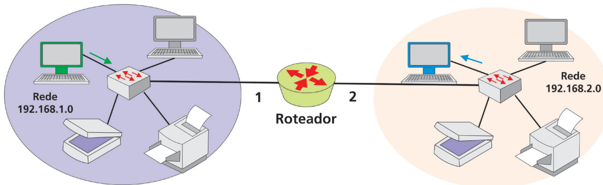
Figura 8.10 Roteamento de pacotes Fonte: adaptado de Olifer (2008)
