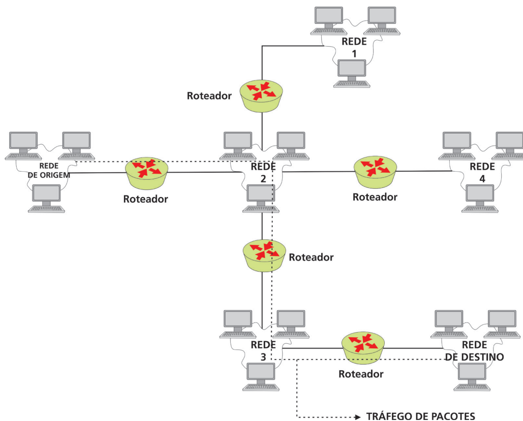
Figura 8.11 Interligação de redes com roteadores
