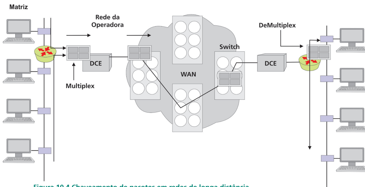
Figura 10.4 Chaveamento de pacotes em redes de longa distância
