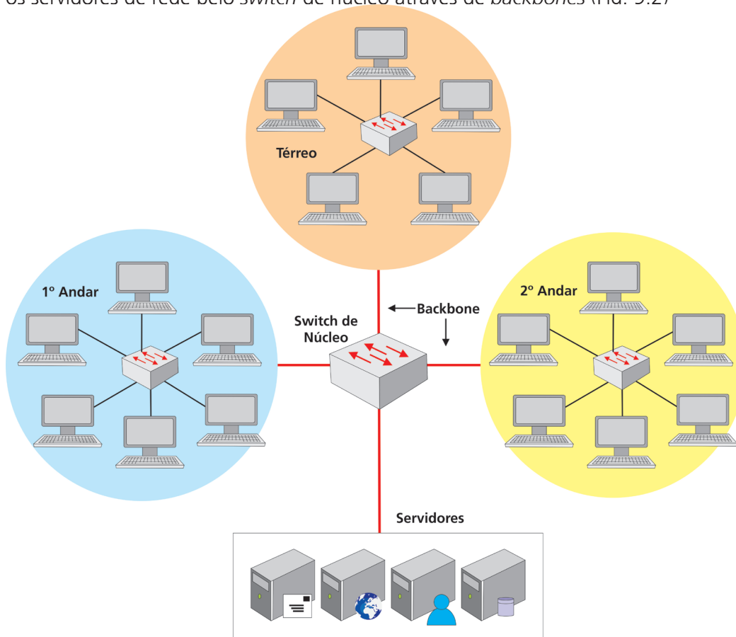
Figura 9.2 Topologia de redes locais
