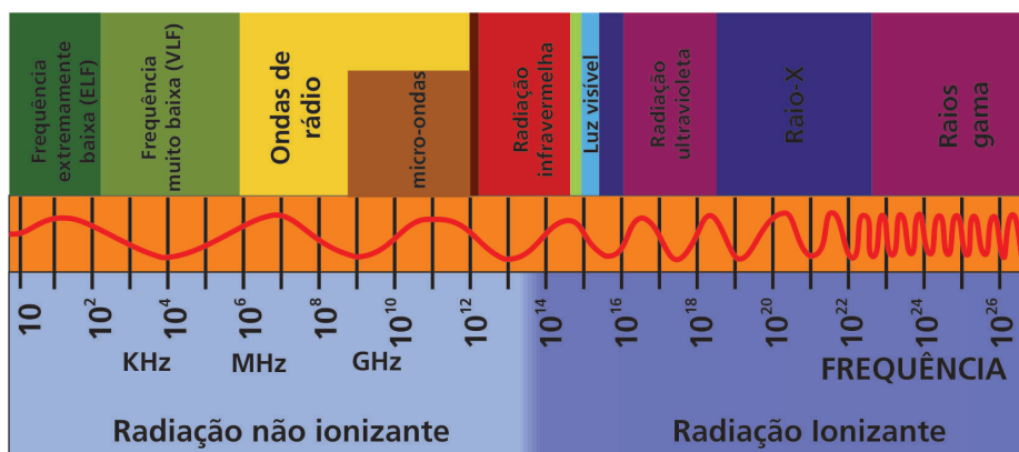
Figura 3.6 Espectro eletromagnético
