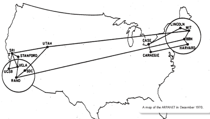
Figura 6.1 Mapa da Arpanet em dezembro de 1970
