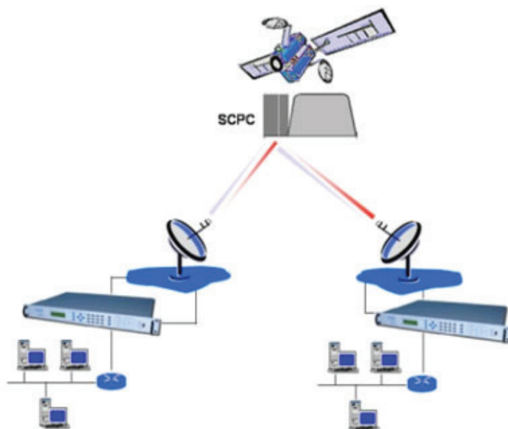
Figura 2.7 Comunicação ponto a ponto
