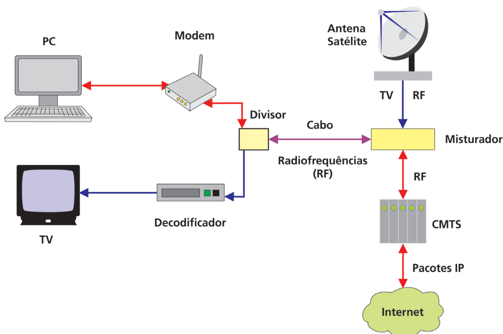
Figura 10.2 Banda larga através de cabo
