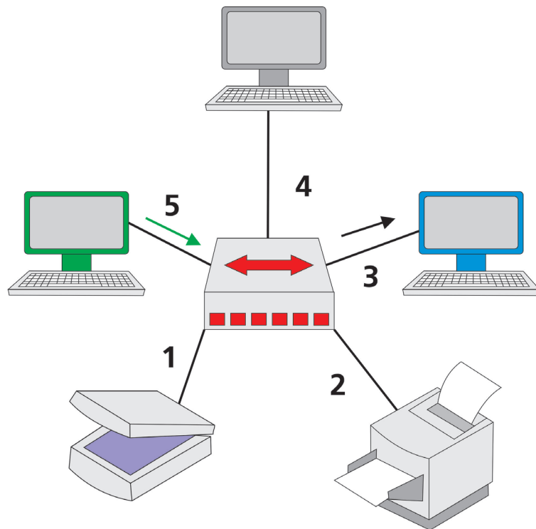
Figura 8.5 Conectividade com comutador
