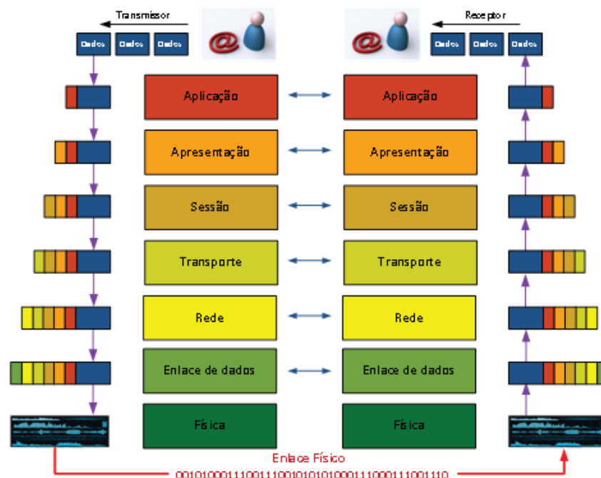
Figura 5.2 Modelo de referência OSI
