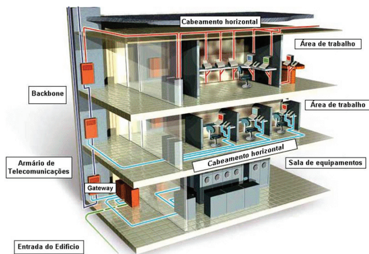
Figura 9.1 Rede local empresarial
